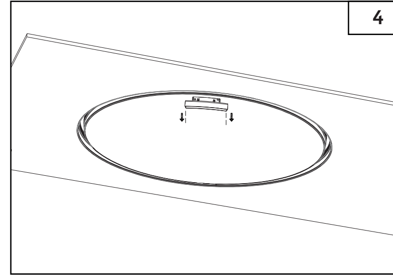
4.1 Armatür gövdesinde bulunan kilit mekanizmasına basılarak armatür kendinize doğru çekilip çıkartılır. 4.1 By pressing the locking mechanism on the fixture body, the fixture is pulled towards you and removed.
