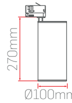
Ağırlık/Weight:1,4 Kg
