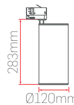
Ağırlık/Weight:1,7 Kg
